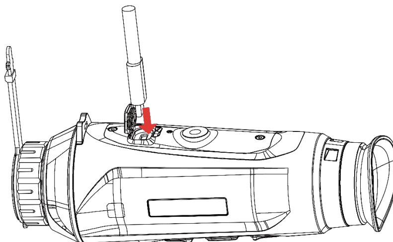
Obrázek 2-4 Zapojení kabelů
