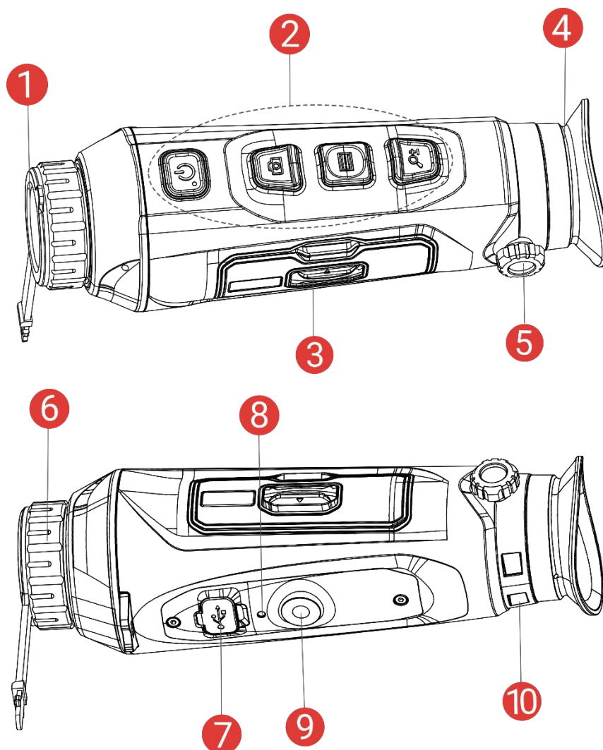
Obrázek 1-1 Vzhled
